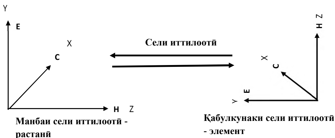
Расми 2. Схемаи принципалии таъсири байнихамдигарии манбаъ ва қабулкунак
